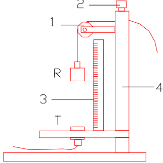
1一定滑轮 2螺栓 3刻度尺 4支架 图 A.0.1 换能器悬挂装置示意图
