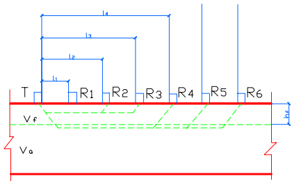
图 8.2.2 检测损伤层厚度示意图
