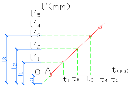
图 5.2.1-1 平测“时-距”图
